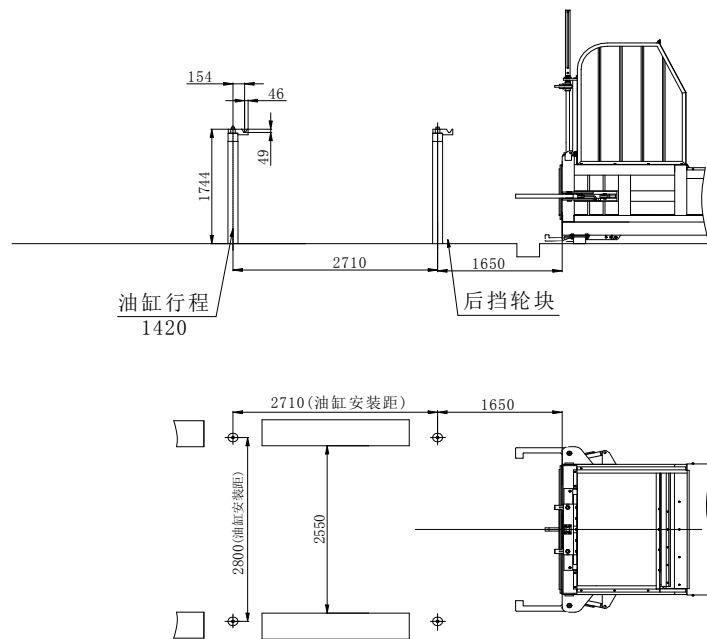
GH250YSJE1型压缩站主要参数示意图
